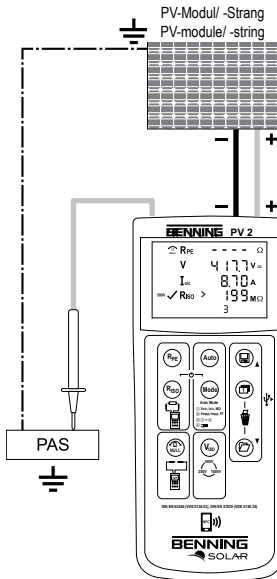
Bild 6: Automatische Solarmodul-Messung, ISO-Messung über Erdleiter Fig. 6: Automatic solar panel measurement, ISO measurement via earthing conductor
