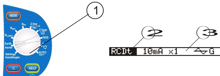
Figuur 14 Draaischakelaar en bijbehorende functieregel
