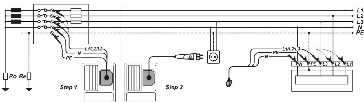
Figuur 7.4: Auto-Test aansluiting
