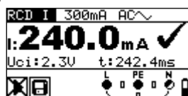
Figuur 34 Voorbeeld meetresultaat uitschakelstroom
