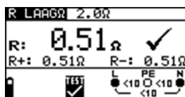
Figuur 22 Voorbeelden van meetresultaten van de weerstand R_{LAAG}
