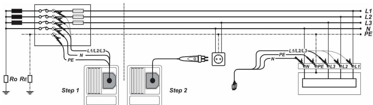
Figuur 6.1: Fase-Nul of Fase-Fase spanningsval meting – via de plug commander en losse aansluitsnoer.
